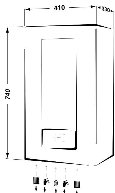
Размеры котла Пантера
