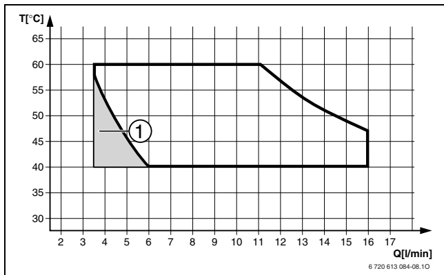
Рис. 12 Діаграма для холодної води на вході від +15^{\circ}\text{C} (ZWC 35-3 MFA)
