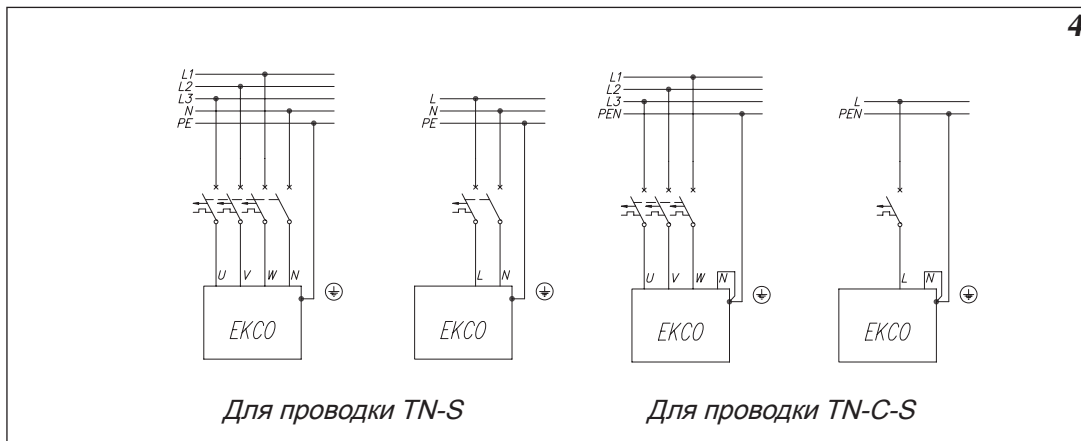
Рис.4 Подключение к электросети
