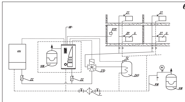
Рис.6 Совместная работа приоритетного котла с котлом ЕКСО
