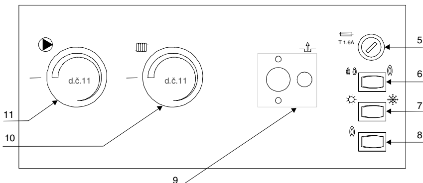
Рис.36 Панель управления вертикальная
