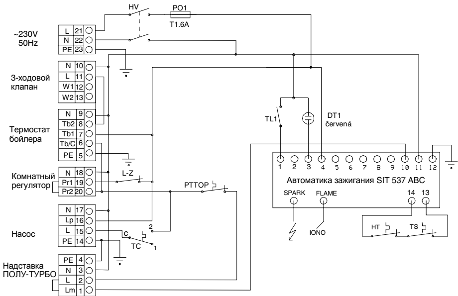
Рис. 46 – Схема электрического подключения 60 KLO
