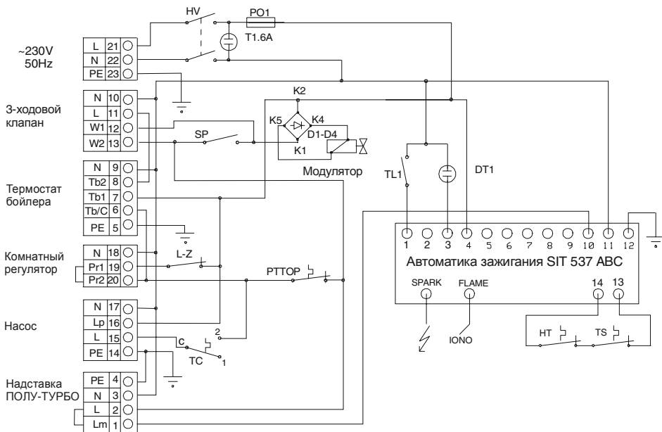
Рис. 4а – Схема электрического подключения 20,30,40,50 KLO
